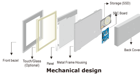
IP65(6mm front bezel)
